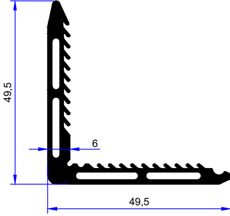
PROFİL KODU / PROFILE CODE 2383 AĞIRLIK / WEIGHT 0,847 GR/M
