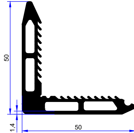
PROFİL KODU / PROFILE CODE 2440 AĞIRLIK / WEIGHT 1,079 GR/M
