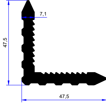
PROFİL KODU / PROFILE CODE 2369 AĞIRLIK / WEIGHT 1,373 GR/M
