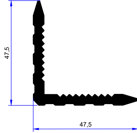
PROFİL KODU / PROFILE CODE 2430 AĞIRLIK / WEIGHT 0,993 GR/M
