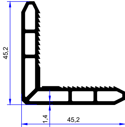
PROFİL KODU / PROFILE CODE 2437 AĞIRLIK / WEIGHT 0,767 GR/M
