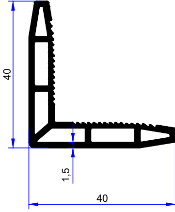
PROFİL KODU / PROFILE CODE 2346 AĞIRLIK / WEIGHT 0,668 GR/M
