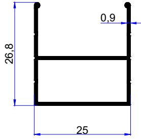
PROFİL KODU / PROFILE CODE 2135 AĞIRLIK / WEIGHT 0,244 GR/M
