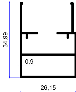
PROFİL KODU / PROFILE CODE 2177 AĞIRLIK / WEIGHT 0,338 GR/M
