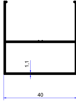
PROFİL KODU / PROFILE CODE 2242 AĞIRLIK / WEIGHT 0,469 GR/M
