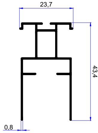
PROFİL KODU / PROFILE CODE 2134 AĞIRLIK / WEIGHT 0,328 GR/M
