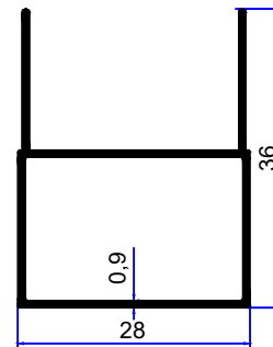
PROFİL KODU / PROFILE CODE 2313 AĞIRLIK / WEIGHT 0,304 GR/M
