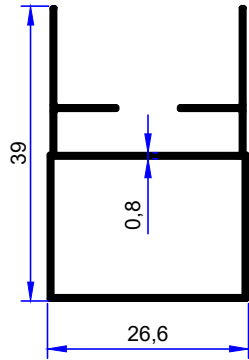
PROFİL KODU / PROFILE CODE 2534 AĞIRLIK / WEIGHT 0,312 GR/M
