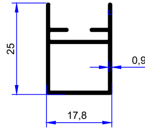
PROFİL KODU / PROFILE CODE 2607 AĞIRLIK / WEIGHT 0,225 GR/M
