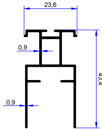
PROFİL KODU / PROFILE CODE 2579 AĞIRLIK / WEIGHT 0,350 GR/M
