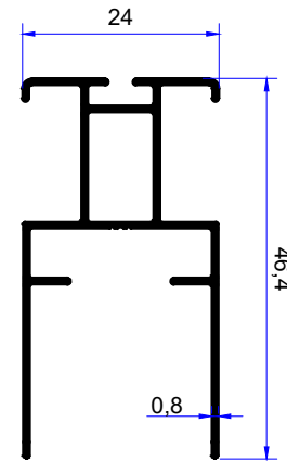
PROFİL KODU / PROFILE CODE 2314 AĞIRLIK / WEIGHT 0,336 GR/M
