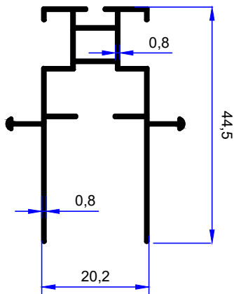
PROFİL KODU / PROFILE CODE 2636 AĞIRLIK / WEIGHT 0,354 GR/M
