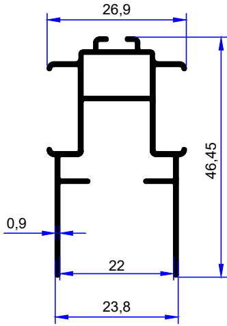
PROFİL KODU / PROFILE CODE 2575 AĞIRLIK / WEIGHT 0,372 GR/M
