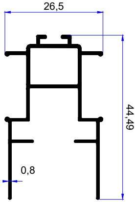
PROFİL KODU / PROFILE CODE 2131 AĞIRLIK / WEIGHT 0,350 GR/M
