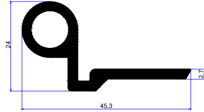
PROFİL KODU / PROFILE CODE 2191 AĞIRLIK / WEIGHT 0,607 GR/M
