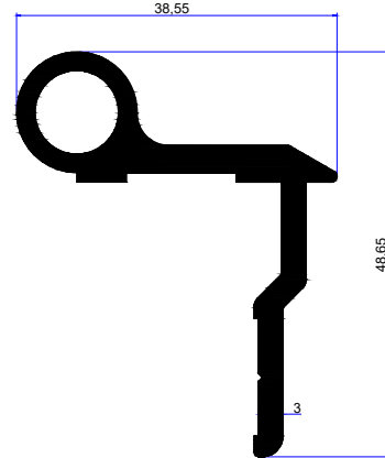
PROFİL KODU / PROFILE CODE 2193 AĞIRLIK / WEIGHT 0,797 GR/M
