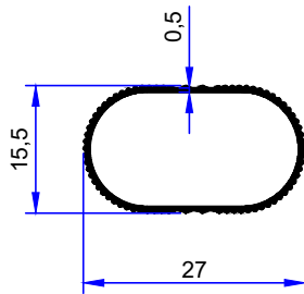
PROFİL KODU / PROFILE CODE 2391 AĞIRLIK / WEIGHT 0,123 GR/M
