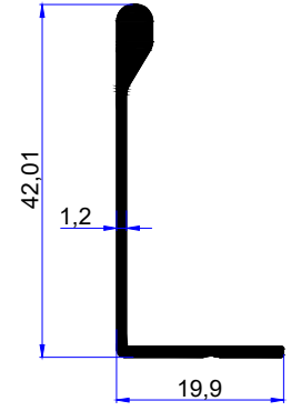
PROFİL KODU / PROFILE CODE 2648 AĞIRLIK / WEIGHT 0,260 GR/M
