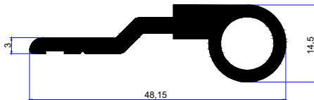
PROFİL KODU / PROFILE CODE 2192 AĞIRLIK / WEIGHT 0,602 GR/M
