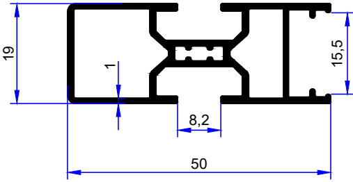
PROFİL KODU / PROFILE CODE 2611 AĞIRLIK / WEIGHT 0,566 GR/M
