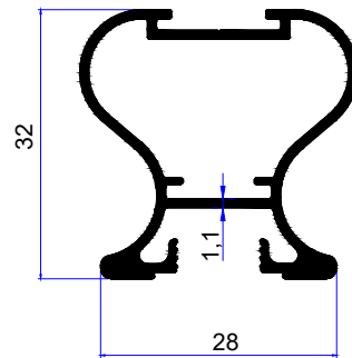
PROFİL KODU / PROFILE CODE 2211 AĞIRLIK / WEIGHT 0,466 GR/M
