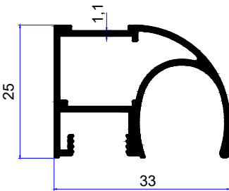
PROFİL KODU / PROFILE CODE 2210 AĞIRLIK / WEIGHT 0,415 GR/M
