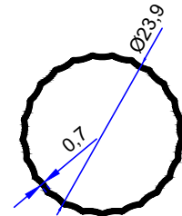
PROFİL KODU / PROFILE CODE 2460 AĞIRLIK / WEIGHT 0,139 GR/M
