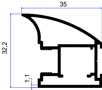
PROFİL KODU / PROFILE CODE 2160 AĞIRLIK / WEIGHT 0,488 GR/M
