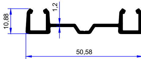
PROFİL KODU / PROFILE CODE 2387 AĞIRLIK / WEIGHT 0,343 GR/M
