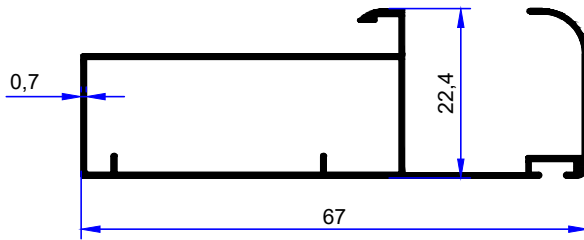
PROFİL KODU / PROFILE CODE 2533 AĞIRLIK / WEIGHT 0,366 GR/M
