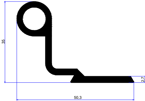
PROFİL KODU / PROFILE CODE 2190 AĞIRLIK / WEIGHT 0,696 GR/M
