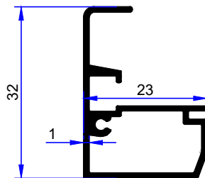
PROFİL KODU / PROFILE CODE 2533 AĞIRLIK / WEIGHT 0,366 GR/M
