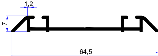
PROFİL KODU / PROFILE CODE 2159 AĞIRLIK / WEIGHT 0,322 GR/M
