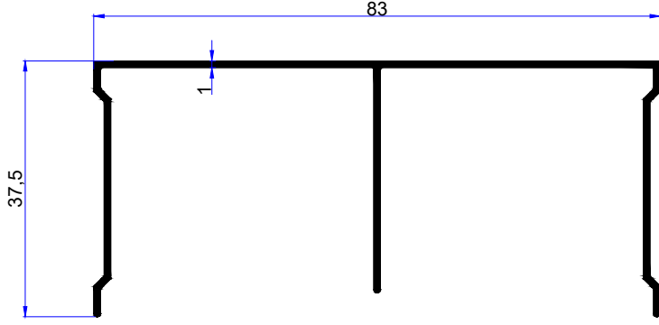
PROFİL KODU / PROFILE CODE 2156 AĞIRLIK / WEIGHT 0,518 GR/M
