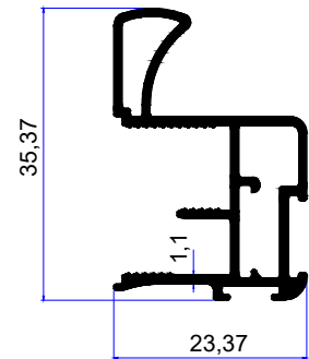
PROFİL KODU / PROFILE CODE 2218 AĞIRLIK / WEIGHT 0,398 GR/M
