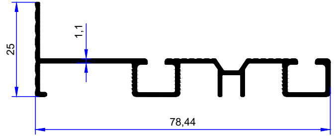
PROFİL KODU / PROFILE CODE 2376 AĞIRLIK / WEIGHT 0,494 GR/M
