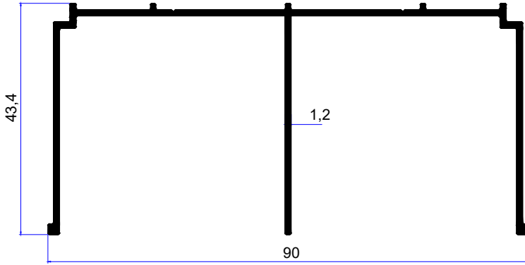
PROFİL KODU / PROFILE CODE 2216 AĞIRLIK / WEIGHT 0,713 GR/M
