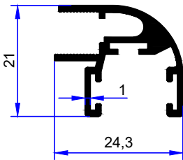
PROFİL KODU / PROFILE CODE 2396 AĞIRLIK / WEIGHT 0,306 GR/M
