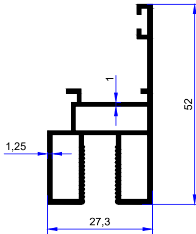
PROFİL KODU / PROFILE CODE 2398 AĞIRLIK / WEIGHT 0,599 GR/M
