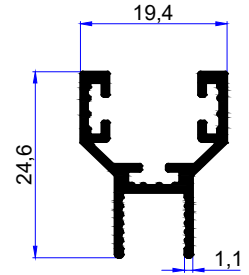
PROFİL KODU / PROFILE CODE 2394 AĞIRLIK / WEIGHT 0,252 GR/M
