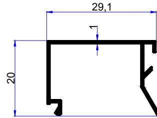
PROFİL KODU / PROFILE CODE 2666 AĞIRLIK / WEIGHT 0,211 GR/M
