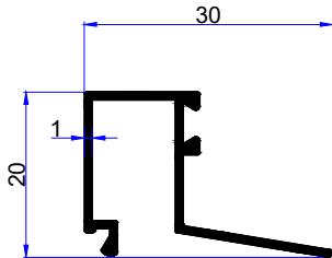
PROFİL KODU / PROFILE CODE 2665 AĞIRLIK / WEIGHT 0,211 GR/M
