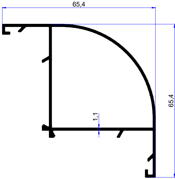
PROFİL KODU / PROFILE CODE 2662 AĞIRLIK / WEIGHT 0,702 GR/M
